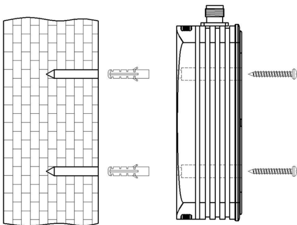
Схема расположения монтажных отверстий (размеры указаны в миллиметрах)
